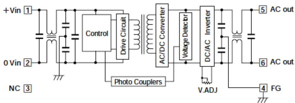
図2.2 ブロック図
